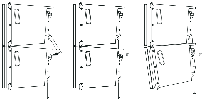
图14. M-FXA 线阵列的前后连接
