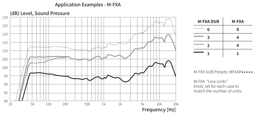
图 53. M-FXA SUB 低音音箱和 M-FXA 音箱在不同组合方式下获得的频响
