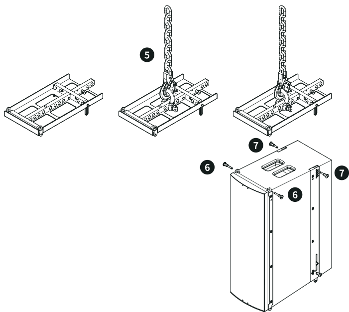
图 16. 连接 M-FXA FS 低音音箱到 M-F3A FS BF 吊架
