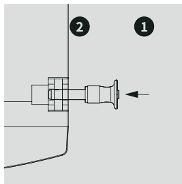
图 6. M-FXA系列产品中安全插销的操作过程
