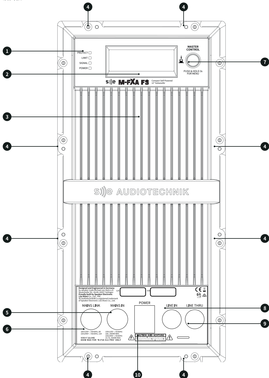
图3. M-FXA SUB 与 M-FXA FS 的后面板
