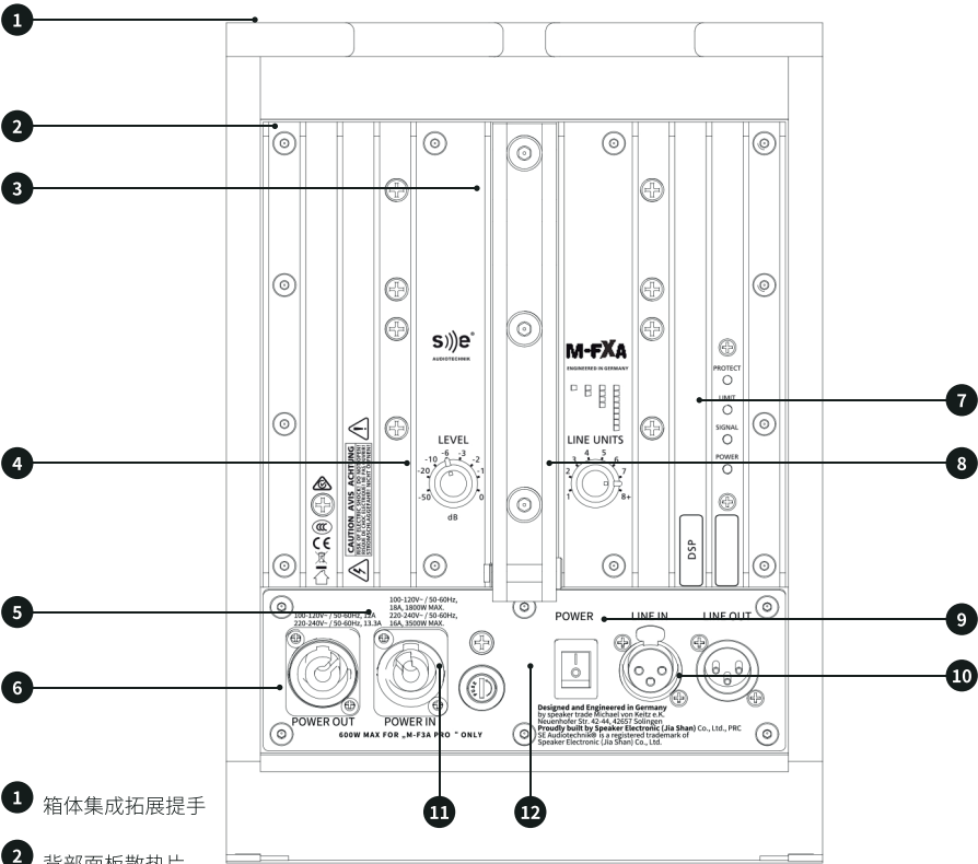
图2. M-FXA 后面板
