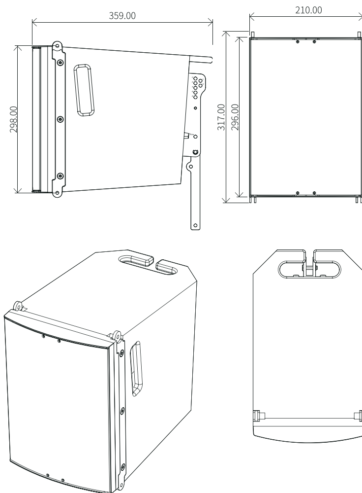
图56.M-FXA 的三视图和尺寸, 注释以毫米为单位。
