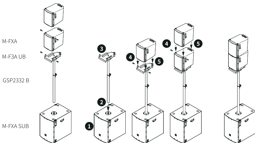
图9. 安装带有 GSP2332 B 支撑杆和 M-F3A UB U 型架的小型阵列。
