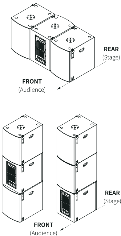
图 54. 心形设置的部分配置
