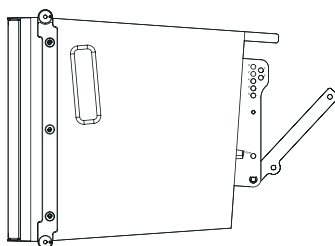
图 5. M-FXA 音箱的前部吊挂点和后部吊挂件
