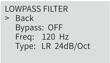
图 31. 低通滤波器调整
