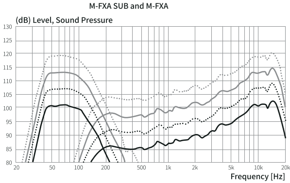
图 51. M-FXA SUB 低音音箱与 M-FXA 音箱在不同组合方式下获得的声压级
