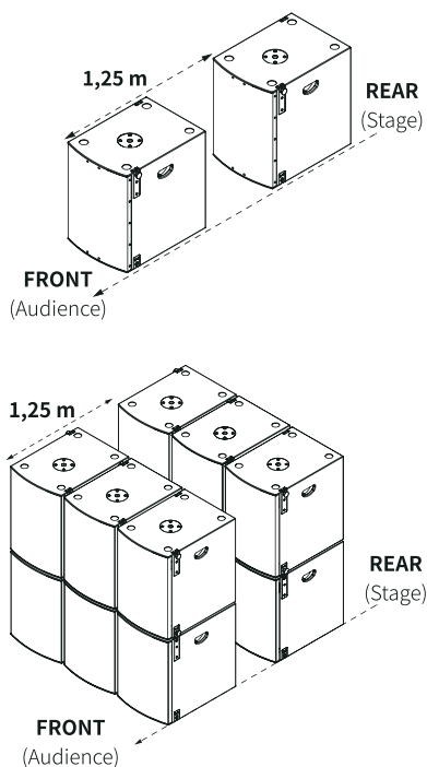
图55. M-FXA SUB低音音箱的端射设置请注意，距离指的是前后排音箱，网罩间的距离。
