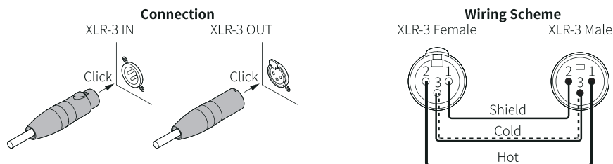
图18. XLR-3接入与串联线缆图示
